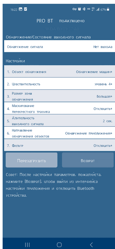
Рис. 7.7. Выбор направления обнаружения
