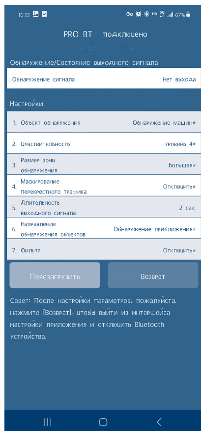
Рис. 7.2. Выбор объекта обнаружения
